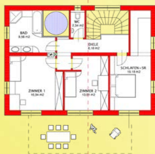
Obergeschoß WNFL 69,81 m 2
